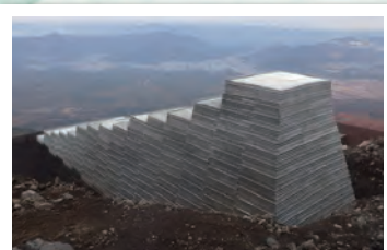
▲登山道導流堤完成状況
